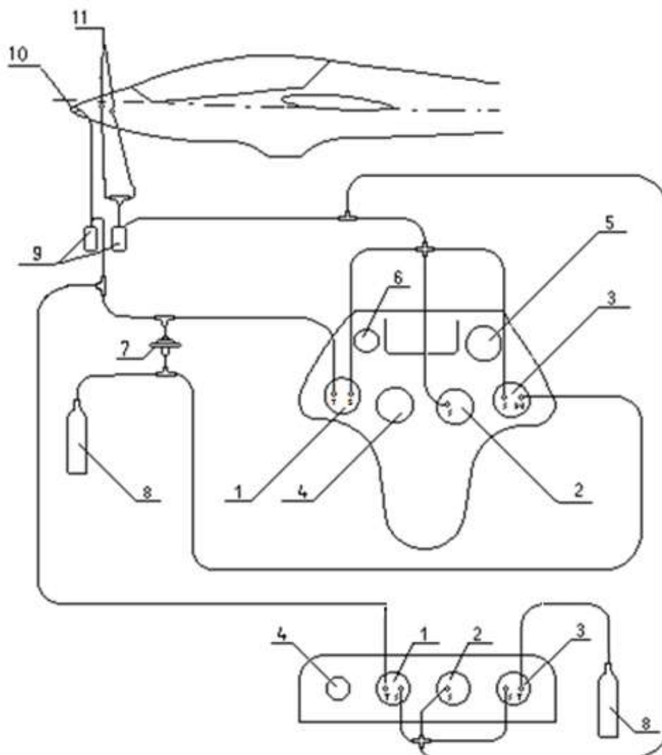
Rys. 7.3 Schemat instalacji ciśnieniowej przyrządów pokładowych.
